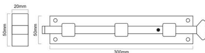
SB-5111-12"
