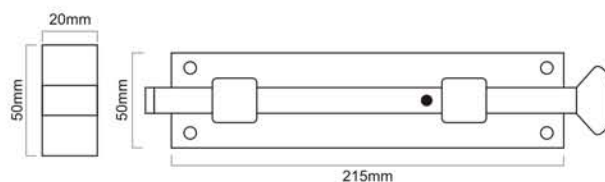
SB-5111-8"
