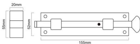
SB-5111-6"
